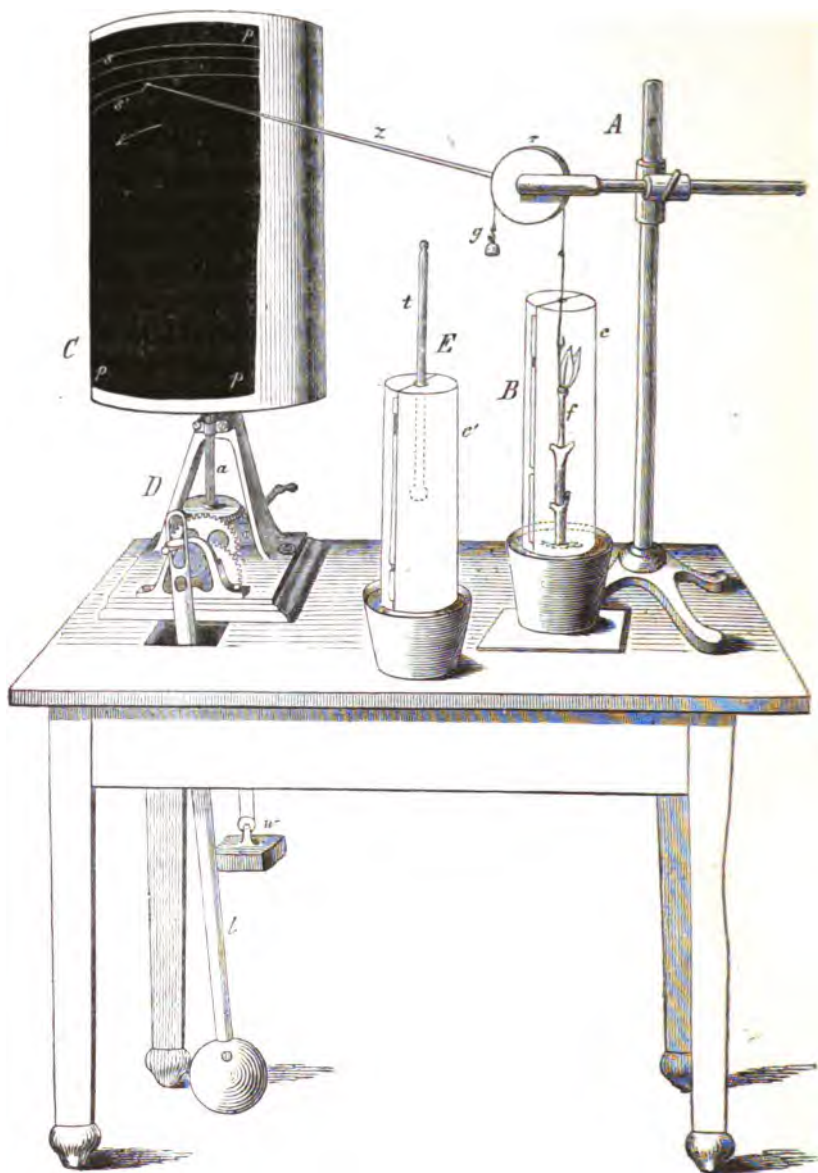
Fig. 450. — Auxanometre enregistreur. Instrument pour mesurer les allongements horaires des entre-nœuds.
